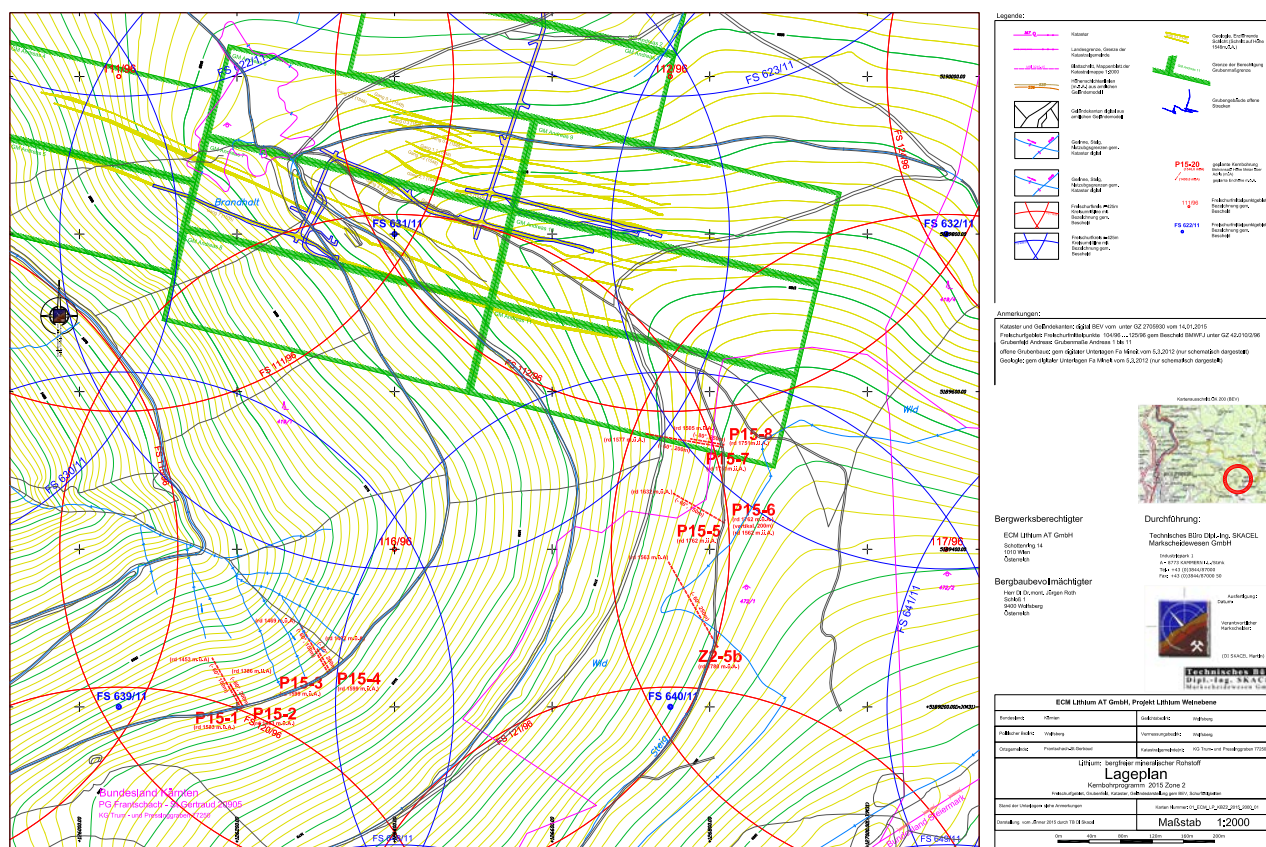
Abbildung 2: Planansicht des Explorationsgebiets in Zone 2 mit den Standorten der Bohrlöcher (rote Nummerierung) im Verhältnis zu den bekannten Erzgängen in Zone 1 im Abbaukonzessionsgebiet (grüne Rechtecke)
