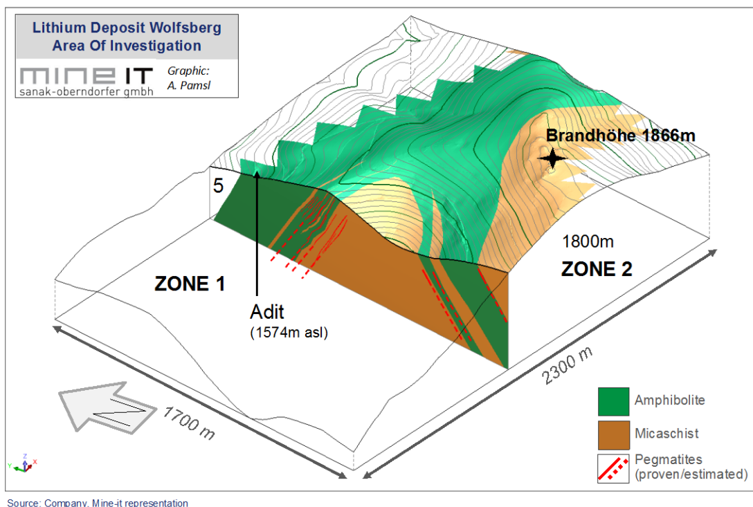
Abbildung 1: Schematische Darstellung der Antiklinale, in der die Erzgänge in Zone 1 sowie potenzielle Erzgänge in Zone 2 zu sehen sind
